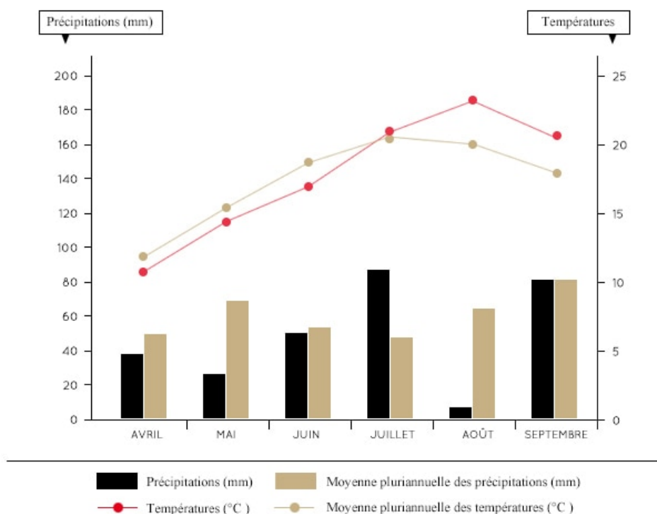
1991 : TEMPÉRATURES ET PRÉCIPITATIONS À SAINT-ÉMILION. COMPARAISON AVEC LES VALEURS NORMALES.
